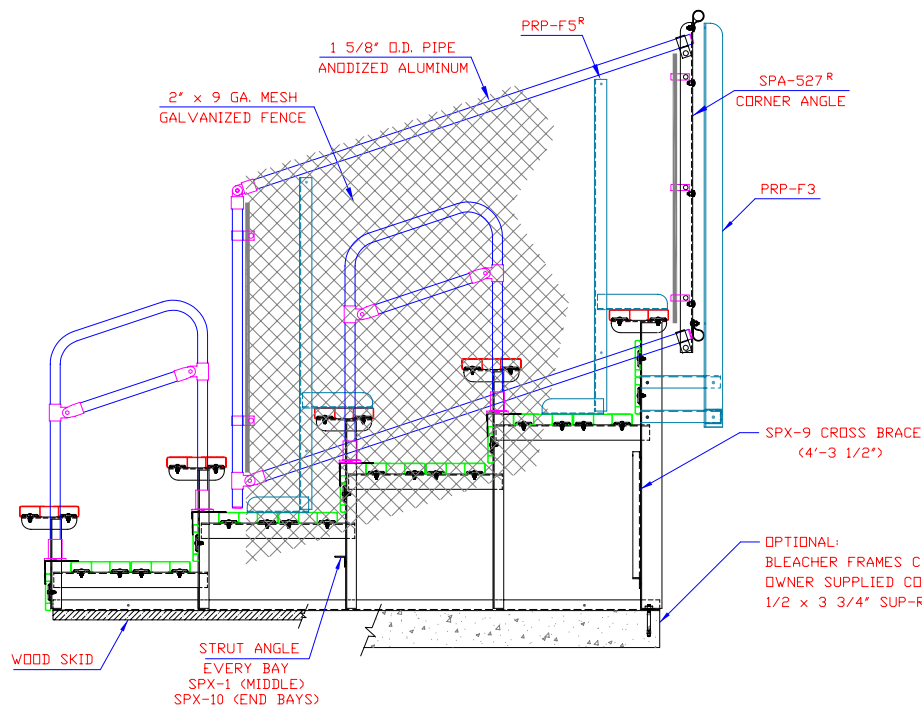
END ELEVATION
