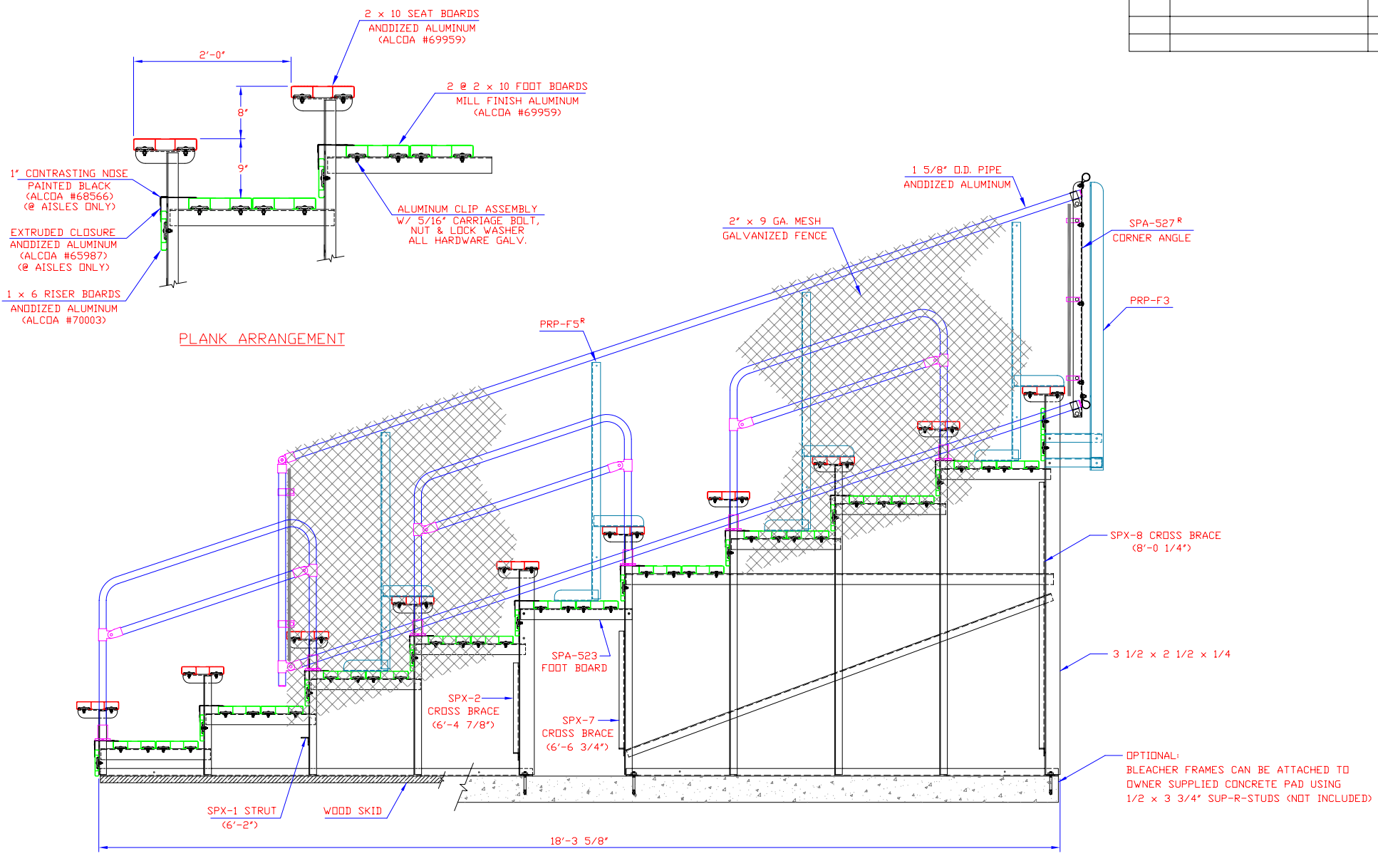
END ELEVATION
