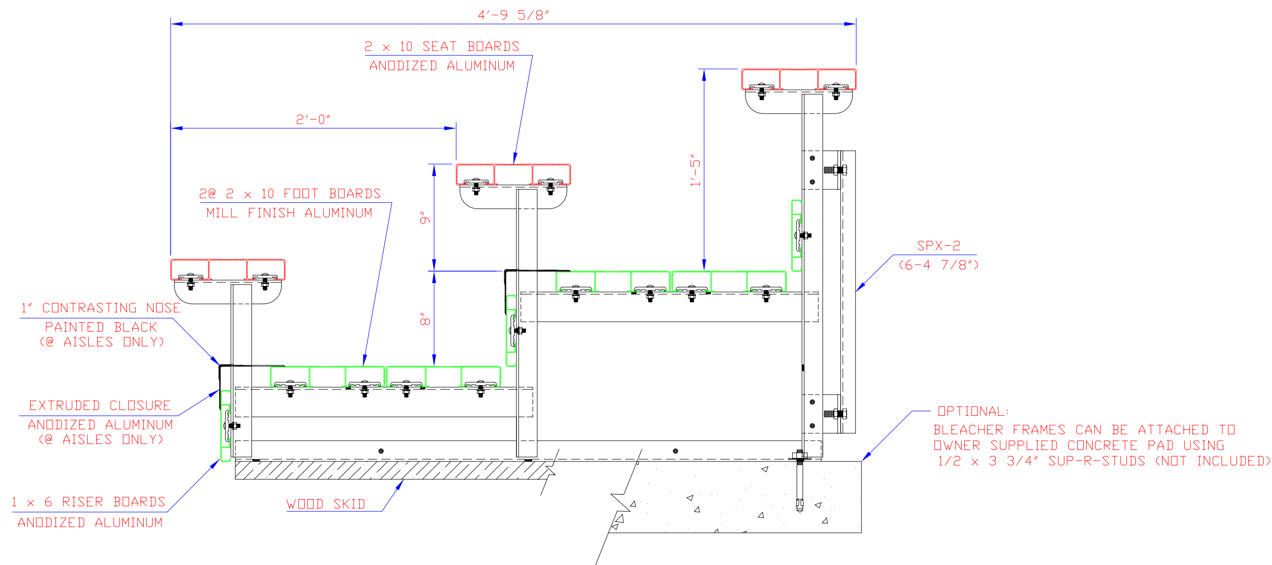
END ELEVATION
