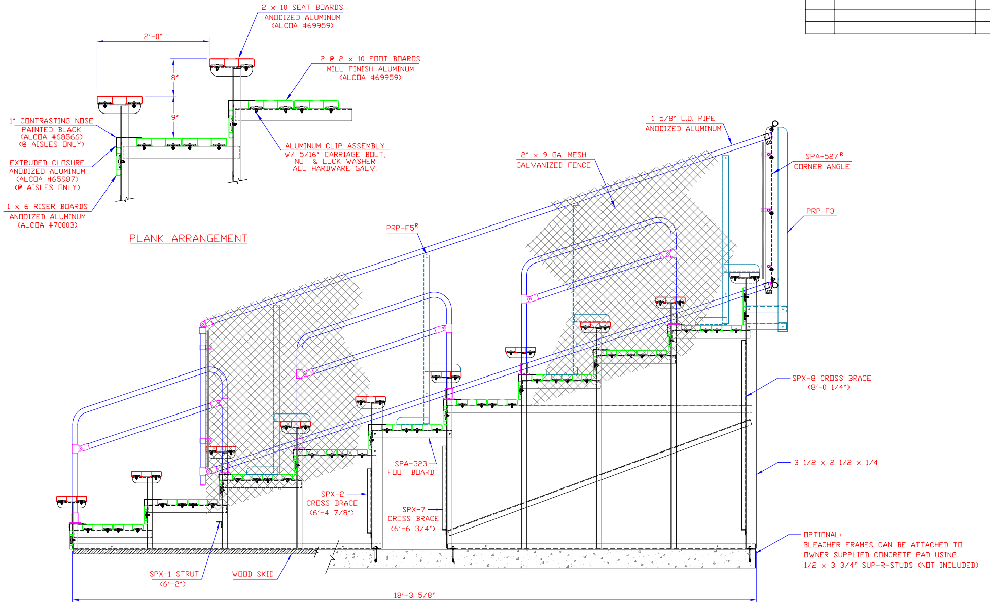
END ELEVATION
