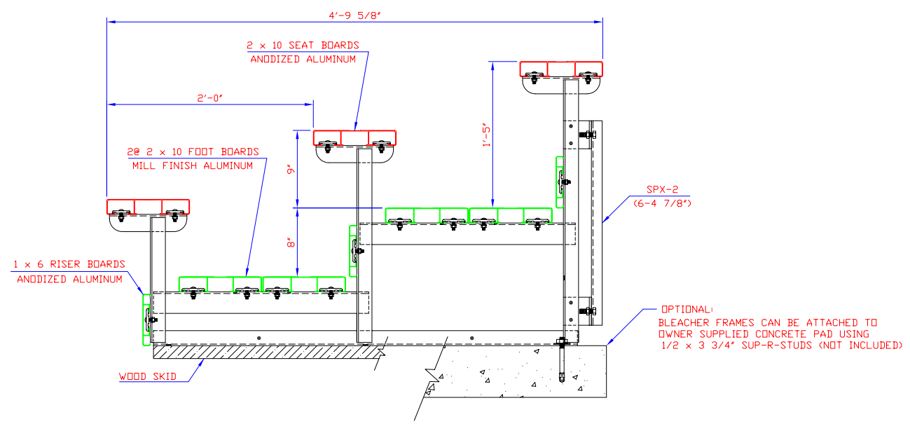
END ELEVATION
