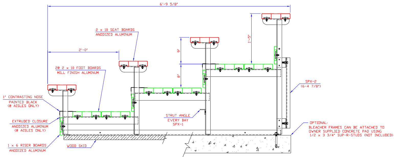
END ELEVATION
