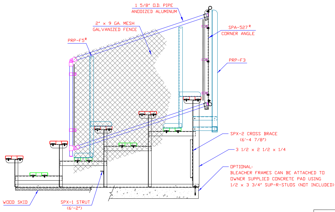
END ELEVATION
