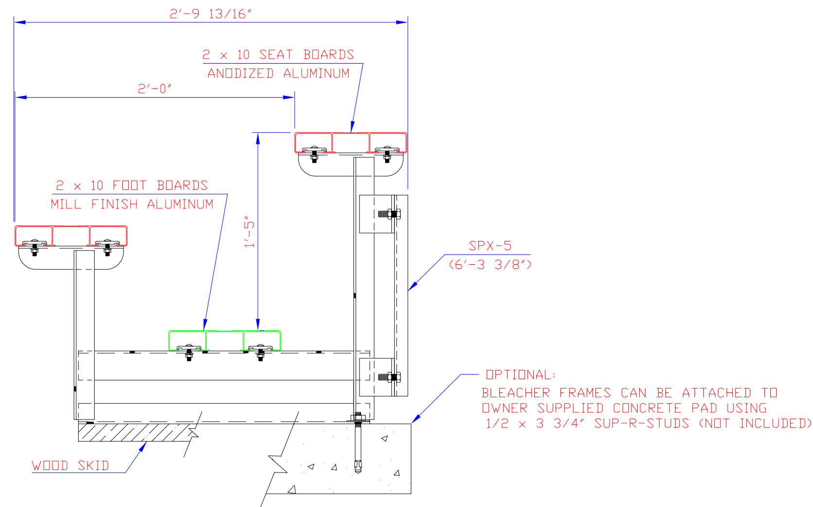
END ELEVATION
