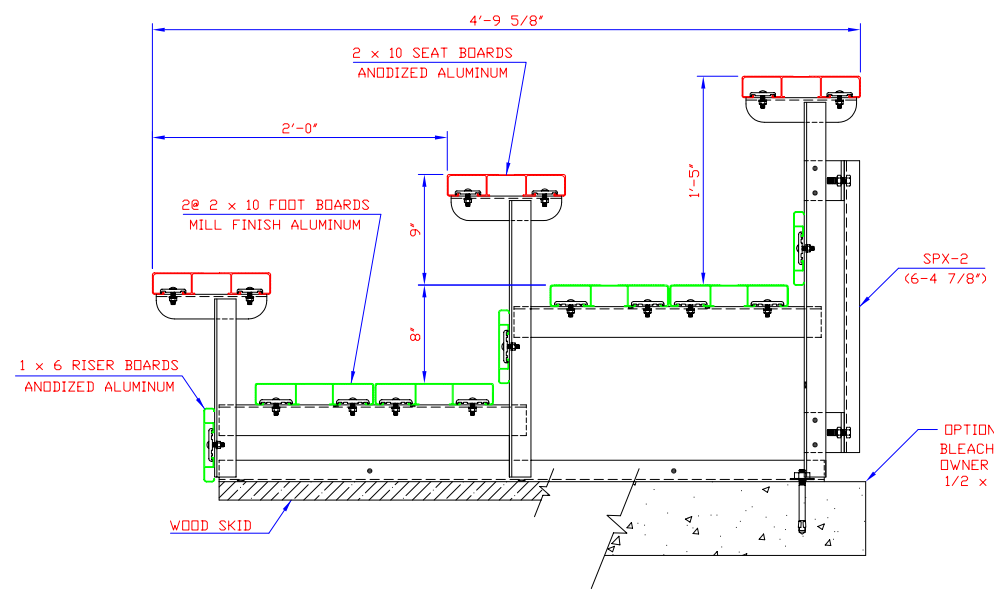
END ELEVATION
