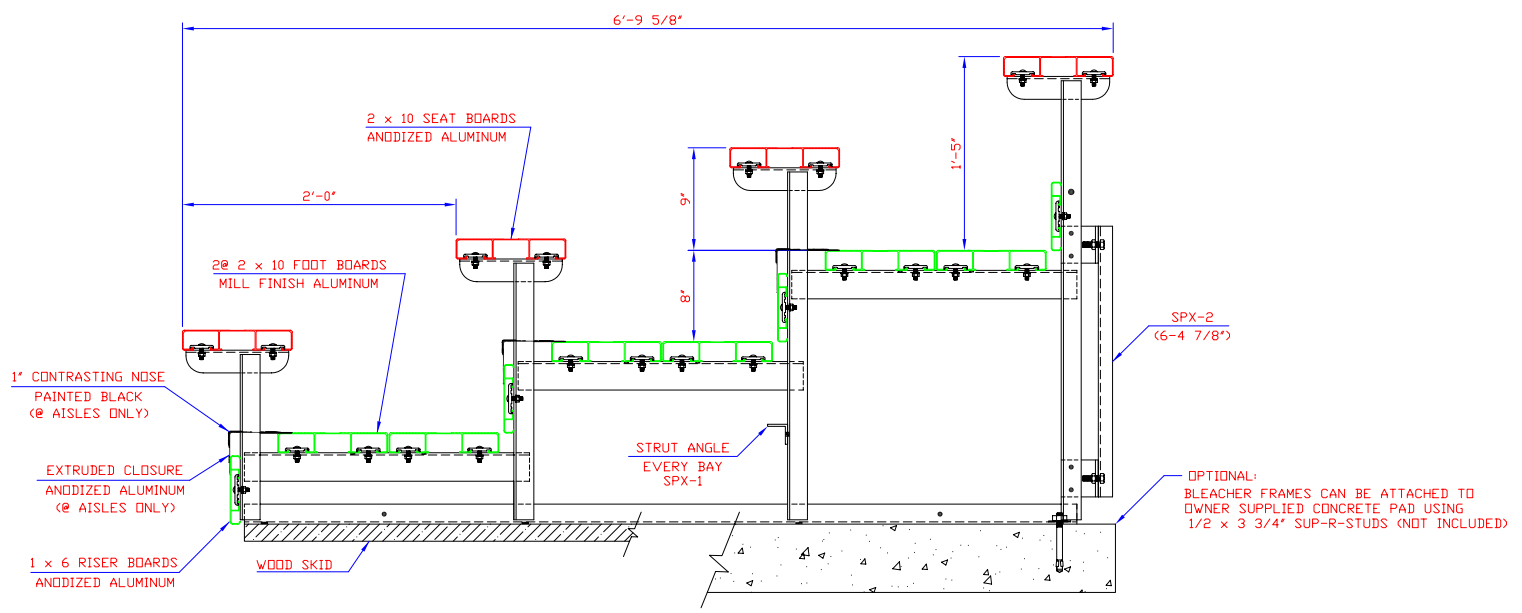
END ELEVATION
