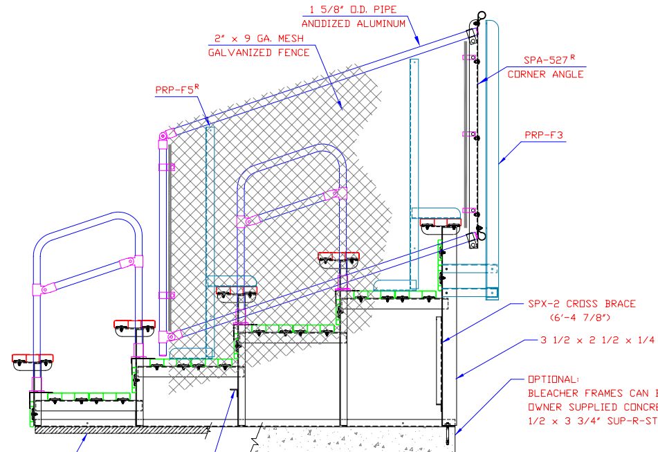
END ELEVATION
